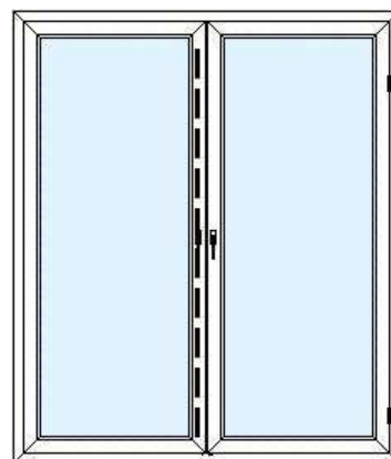
Type U9 - indadgående Med dreje/kip åbning PVC bundstykke
