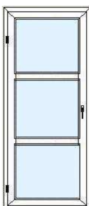
Type U18 Ind/udadgående Med aluminiums bundstykke
